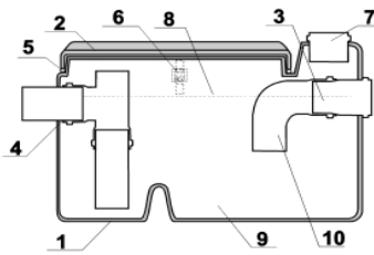
Принципова схема жирословлявача серії СЖ "Оптима"
